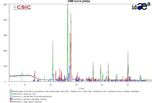
2.-Difractograma de la sorra de platja.
