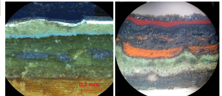
Micrografies de fusteria (esquerra) i de serralleria (dreta) a més augments (de 40 a 80) necessàries per apreciar les diferents capes i el seu color.
