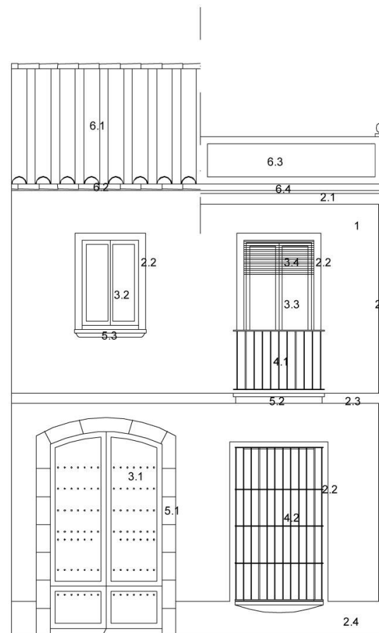
Tipologia de Casa de Cos: Elements que poden contenir de manera aïllada o simultàniament (E:1/75).
